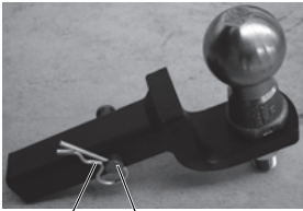
Kupplungsbolzen Federstecker
